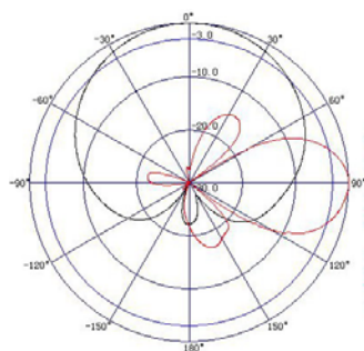
698~960MHz: VPol.
