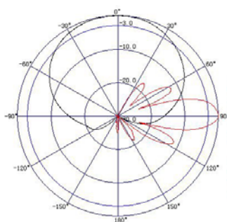
1710~2170MHz: VPol.
